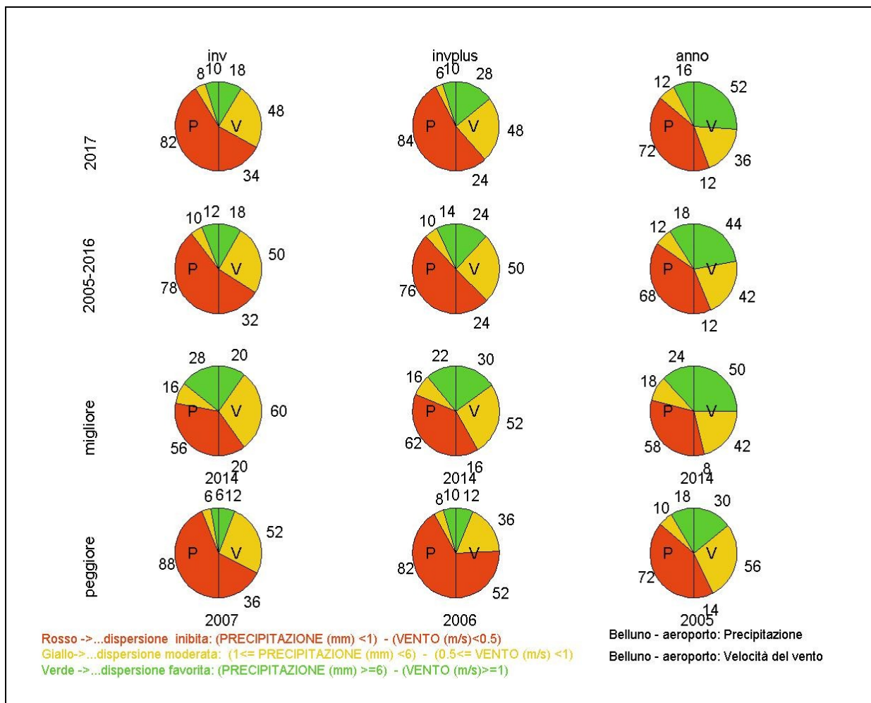
Figura 3: diagrammi circolari per la valutazione sintetica della qualità dell'aria, relative ai mesi invernali, ai mesi invernali + marzo e ottobre (invplus) e annuali, per l'anno 2017, per i corrispondenti periodi più favorevoli alla dispersione (migliore) e meno favorevoli alla dispersione (peggiore) e per la media climatologica (2005-2016), relativamente alla stazione di Belluno Aeroporto.
