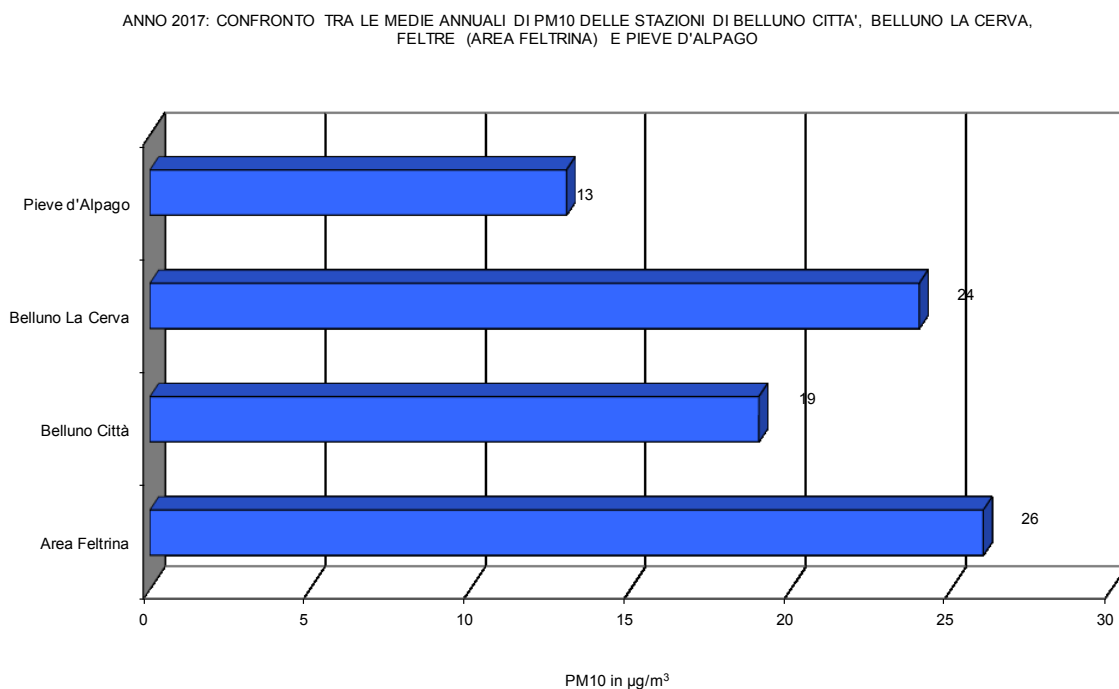
Figura 54: rete di monitoraggio provinciale: medie annuali PM10.
