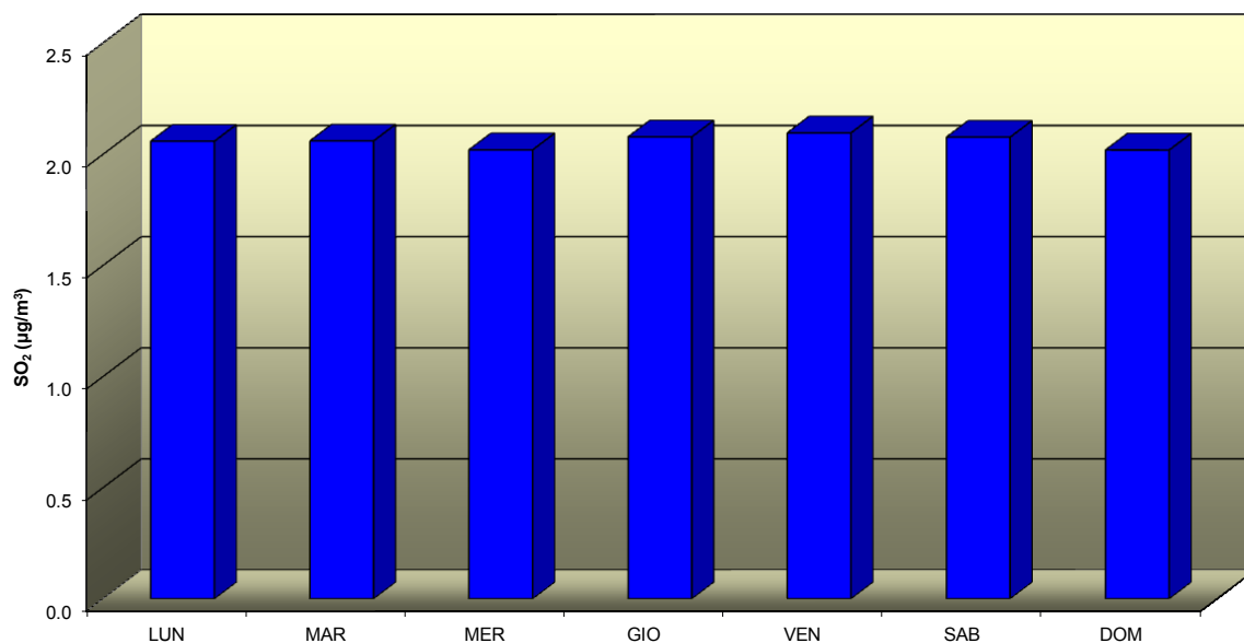
Figura 21: stazione di Belluno; settimana tipo SO 2 .
